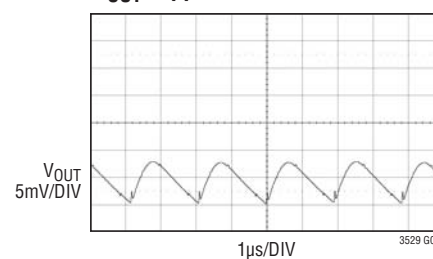
V_{OUT} Ripple
